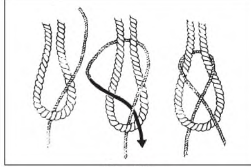
চিত্র : শিট বেণ্ড
